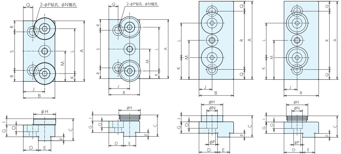
钳口套装75 (扁平型)
