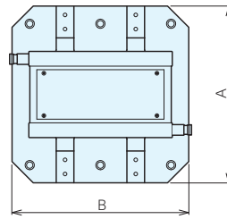
带电磁吸盘MC工作台
