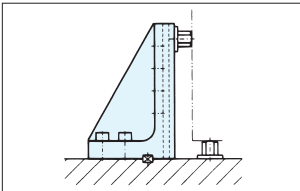
导位块
