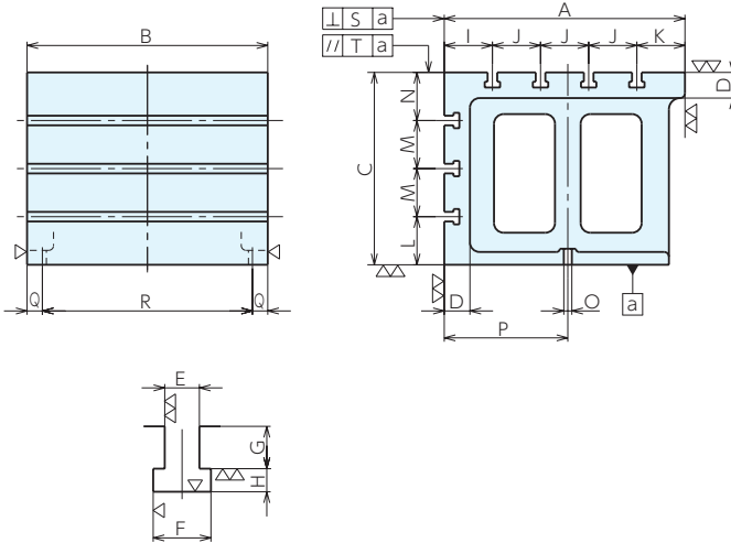
T型槽详图
